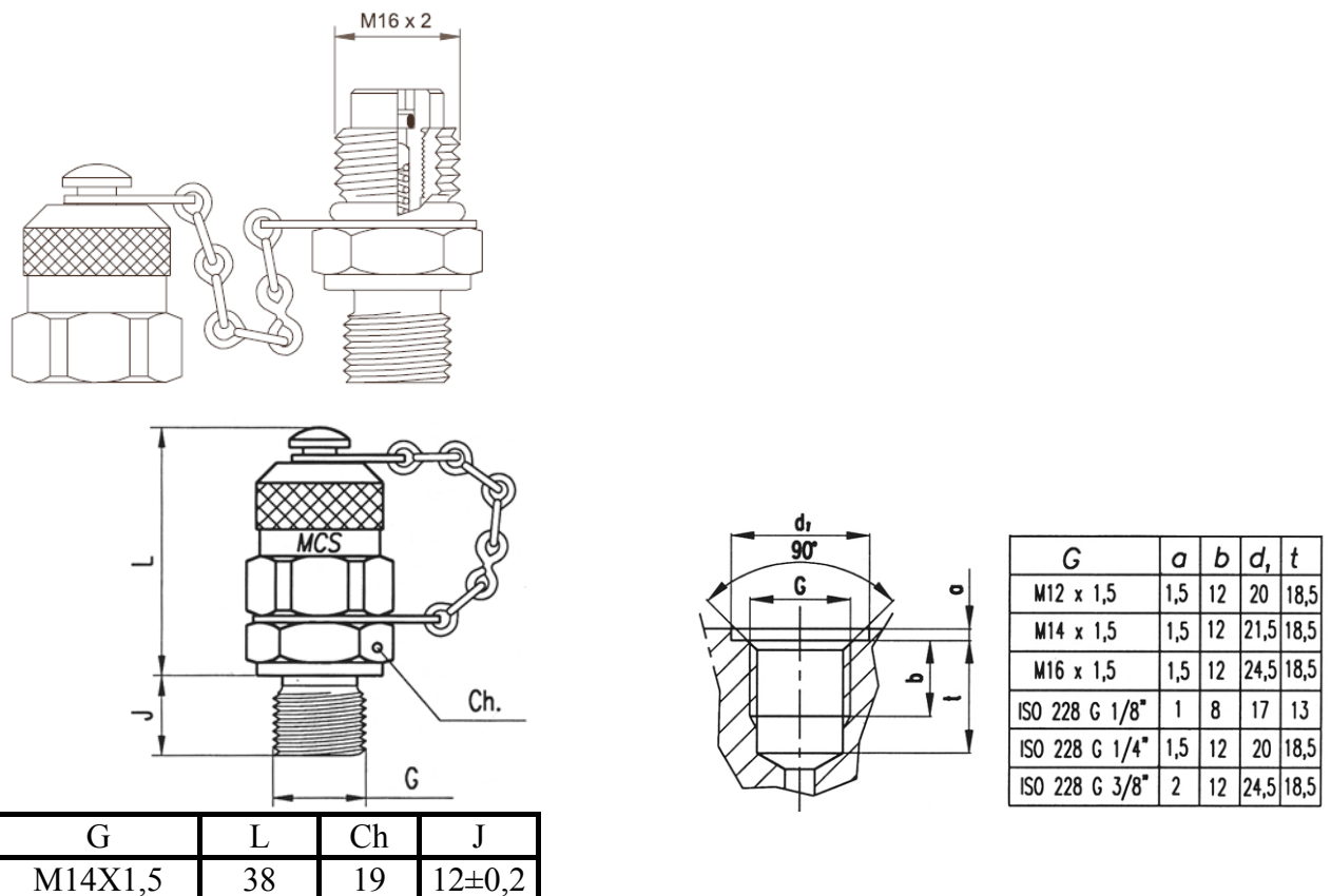
Рис.1. Габаритные и присоединительные размеры ниппель-манометра М14Х1,5 (620.01.014.21) и отверстия под его установку
